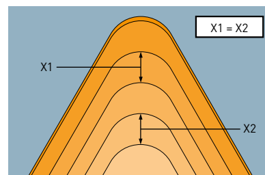
Konstante Schnitttiefe
